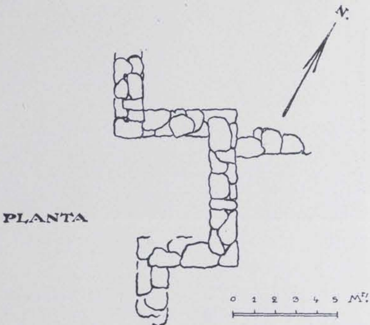
Fig. 81.—Planta d'una de les torres de la muralla de Burriac (per M. Ribes)
